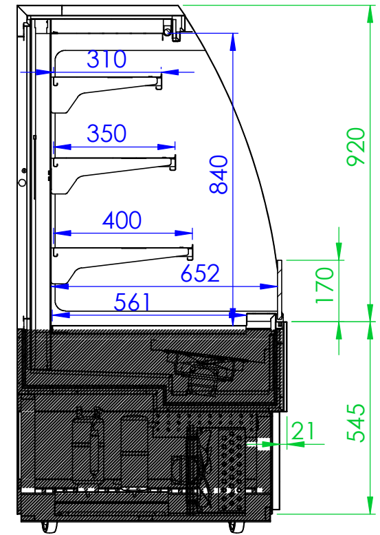
SEZIONE C-C
