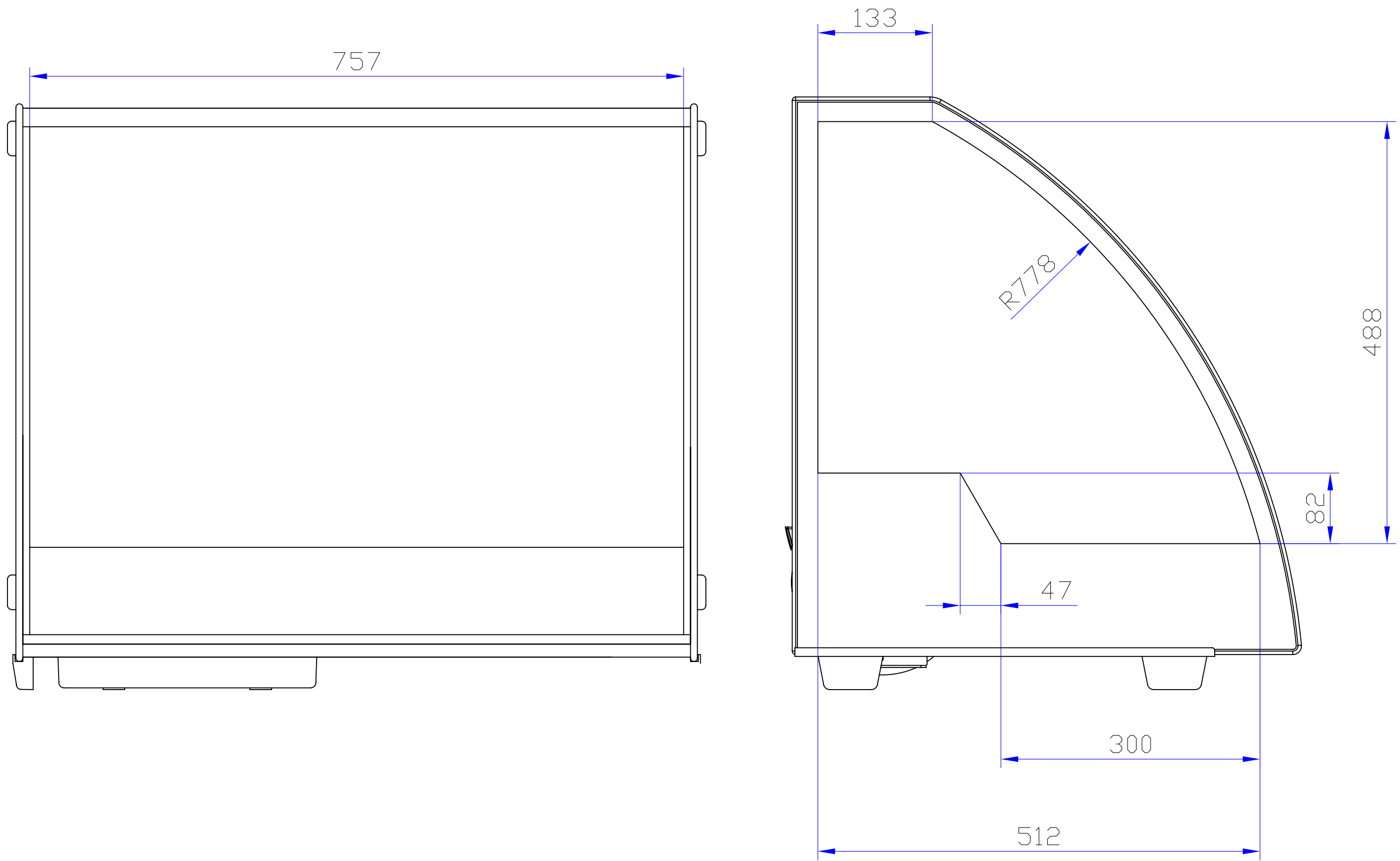
RTW-130L-2内部尺寸图
