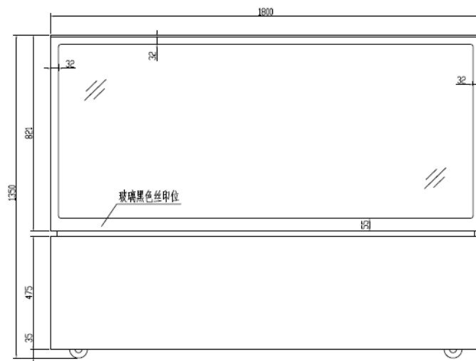
ELEVATION 前视图
