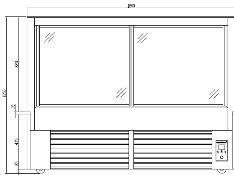
BACK 后视图
