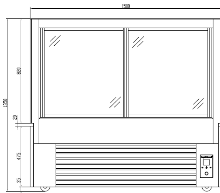
BACK 后视图
