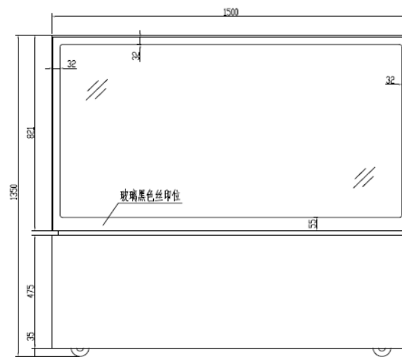
ELEVATION 前视图
