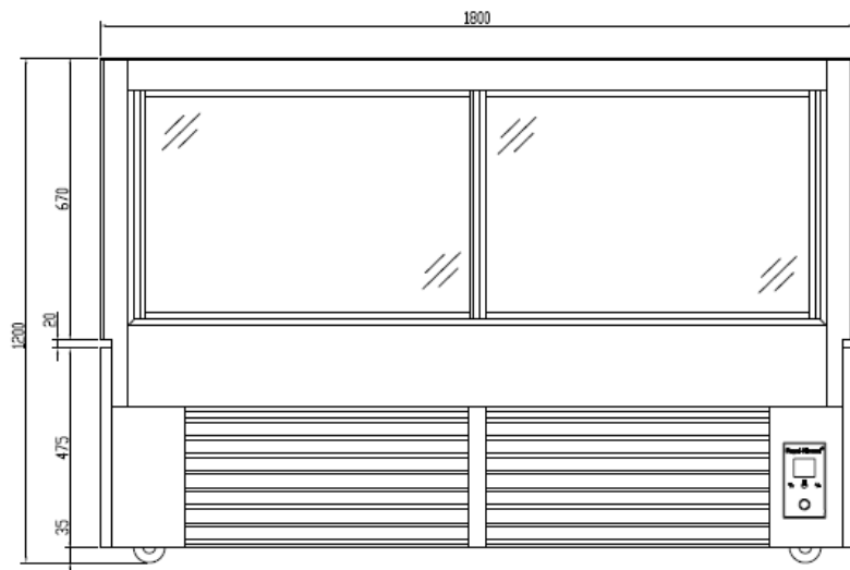
BACK 后视图
