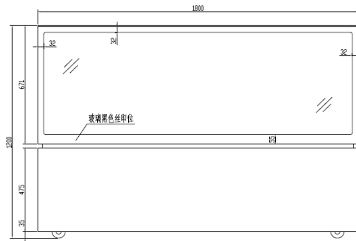
ELEVATION 前视图
