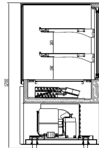
SECTION VIEW 左侧剖视图
