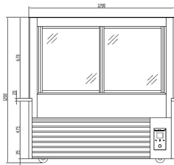
BACK 后视图
