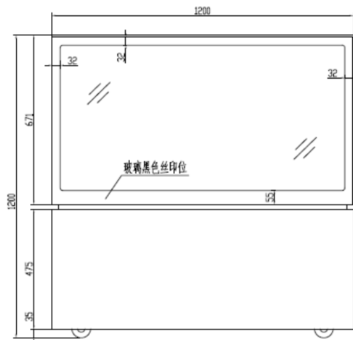
ELEVATION 前视图
