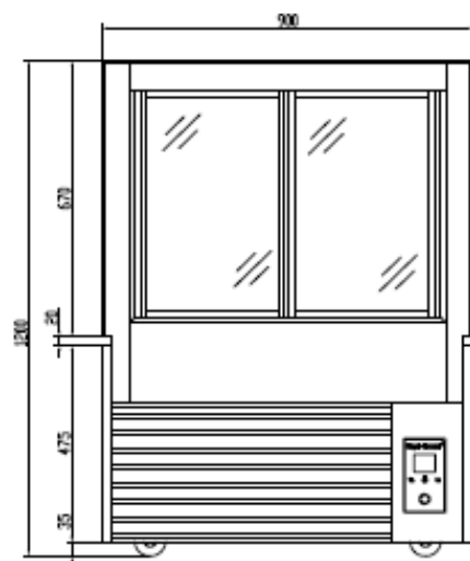
BACK 后视图
