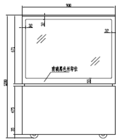
ELEVATION 前视图
