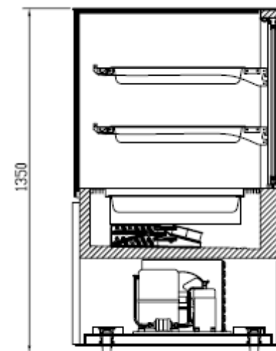
SECTION VIEW 左侧剖视图
