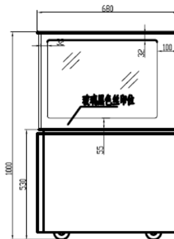
SIDE VIEW 左视图
