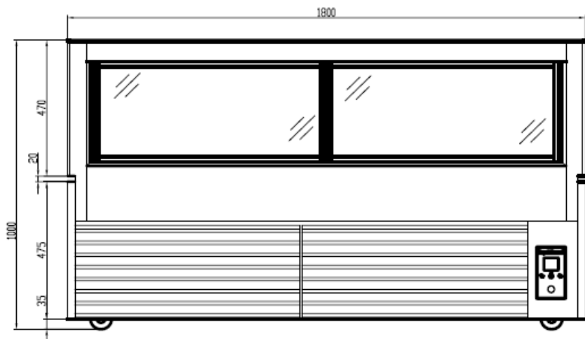
BACK 后视图
