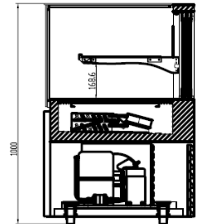
SECTION VIEW 左侧剖视图
