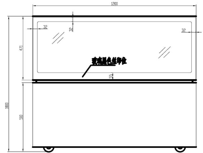
ELEVATION
