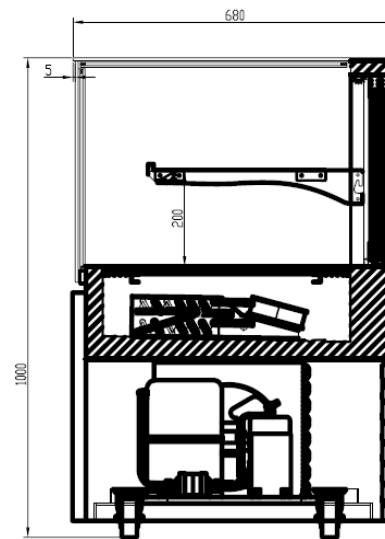
SECTION VIEW 左側剖視圖
