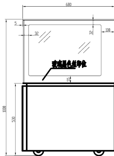
SIDE VIEW 左側視圖
