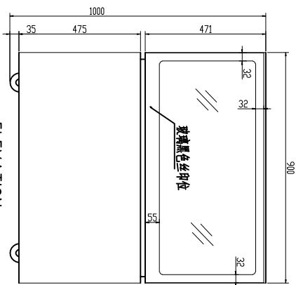
ELEVATION 前视图
