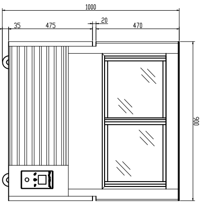
BACK 后视图
