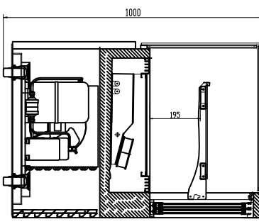
SECTION VIEW 左侧剖视图
