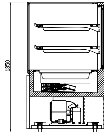
SECTION VIEW 左侧剖视图
