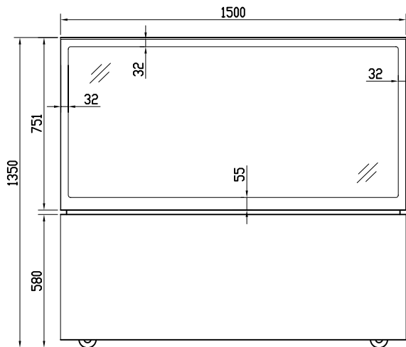
ELEVATION 前视图
