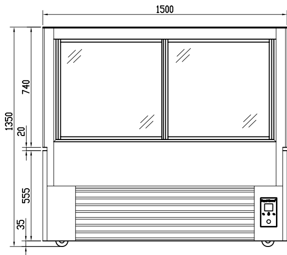
BACK 后视图
