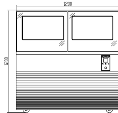
BACK 后视图
