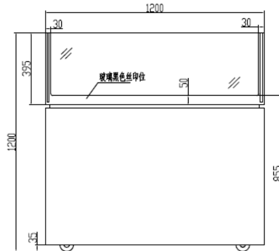
ELEVATION 前视图
