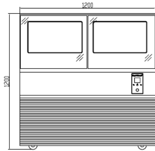
BACK 后视图
