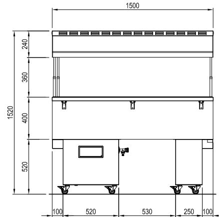
ISOLA INOX BAIN MARIE 6M
