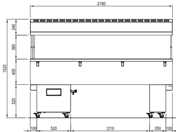
ISOLA INOX BAIN MARIE 6M
